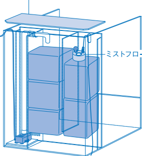
図5 システムテラ 30 背面ろ過フタ
